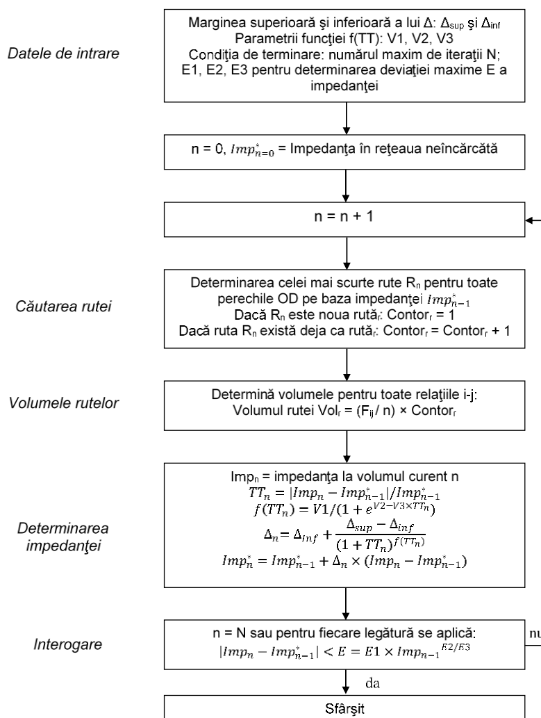
Figură 3-6 Schema logică a metodei "Equilibrium-Lohse" de afectare pe itinerarii
